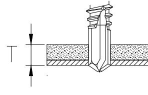
ボード類が硬質で、ボード類にめねじが形成される場合
