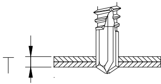
鋼板を重ねた場合
