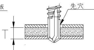
ボード類が硬質で、ボード類にめねじが形成される場合
